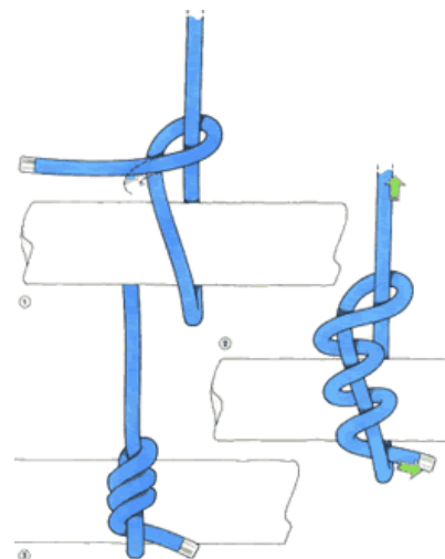
Zimmermannsschlag
