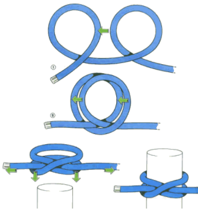
Mastwurf gelegt
